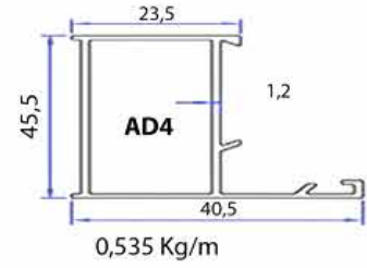
DAR KASA - AL-7103
