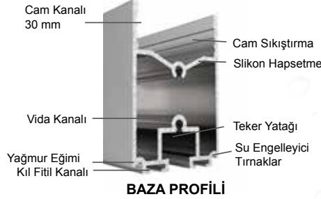
BAZA PROFİLİ
