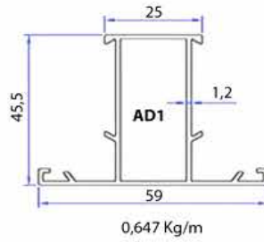
DAR ORTAKAYIT - AL-7104
