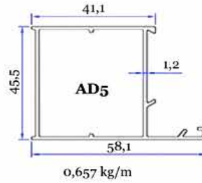
GENİŞ KASA - AL-7108
