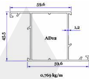
GENİŞ PENCERE KANATLI - AL-7110
