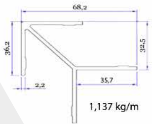
GENİŞ ÇAVUŞ GÖNYE - AL-7107
