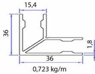
DAR ÇAVUŞ GÖNYE - AL-7102
