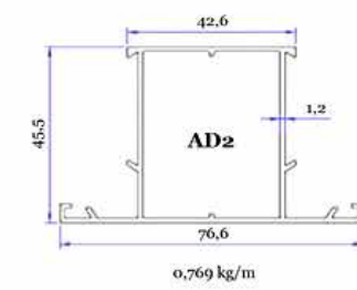
GENİŞ ORTAKAYIT - AL-7109
