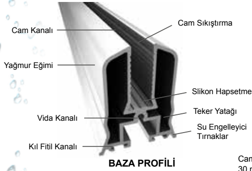
BAZA PROFİLİ
