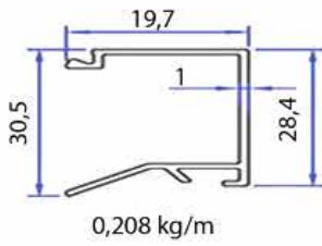
ÇITA - AL-7101
