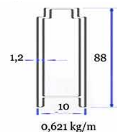
ALM LAMBRI - AL-7112
