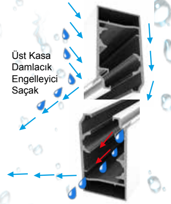
Su Engelleyici Buhar Kanalı
