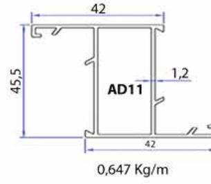
DAR PENCERE KANATI - AL-7105
